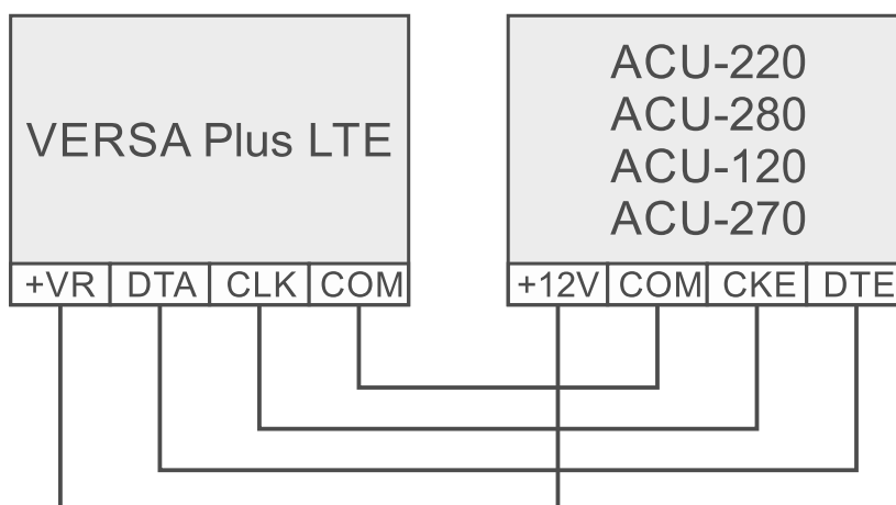
Rys. 7. Sposób podłączenia kontrolera ACU-220 / ACU-280 / ACU-120 / ACU-270 do centrali.
